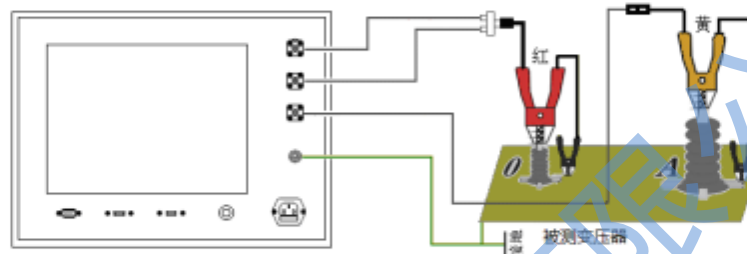
图 2 变压器绕组变形测试的外部接线示意图
