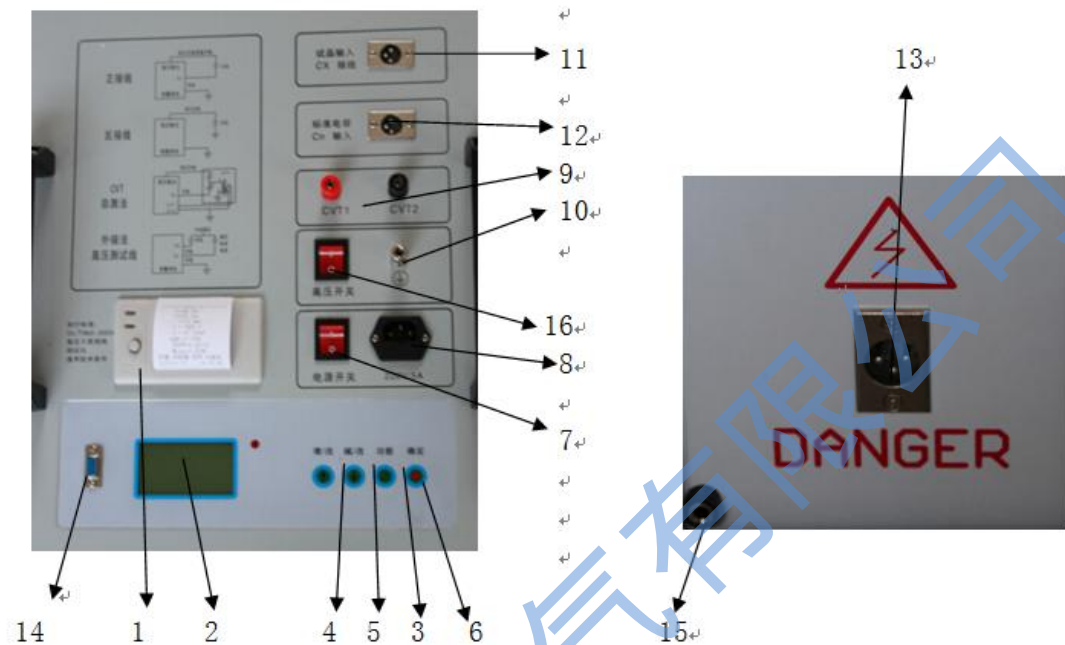
仪器面板图
